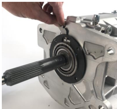
FIG. C REMOVE GASKET
